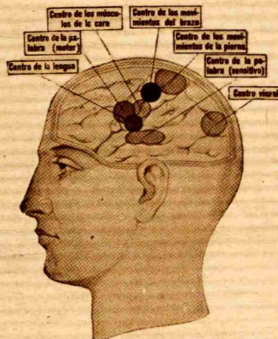
PRINCIPALES CENTROS CEREBRALES
