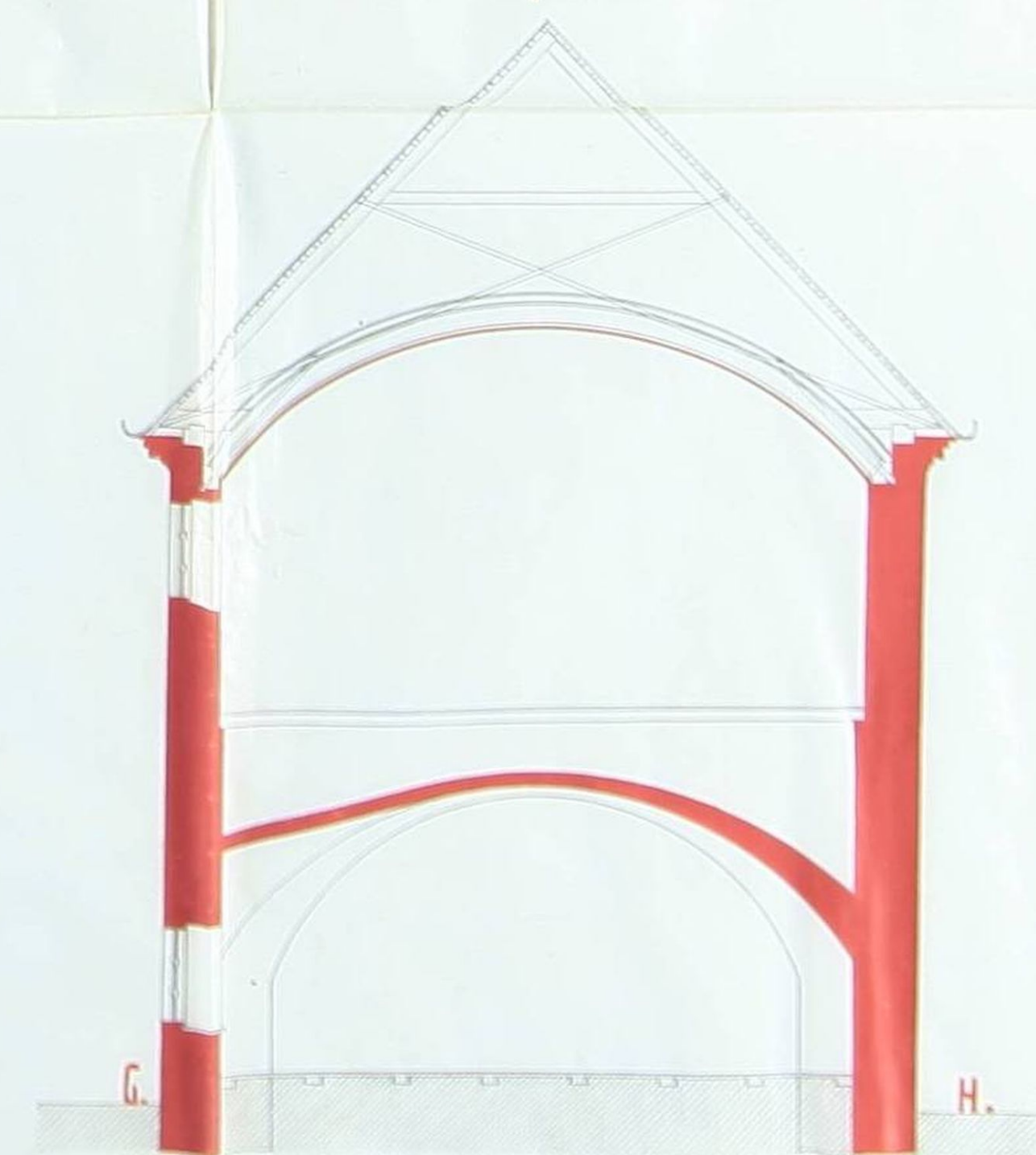
Profil G.H.
