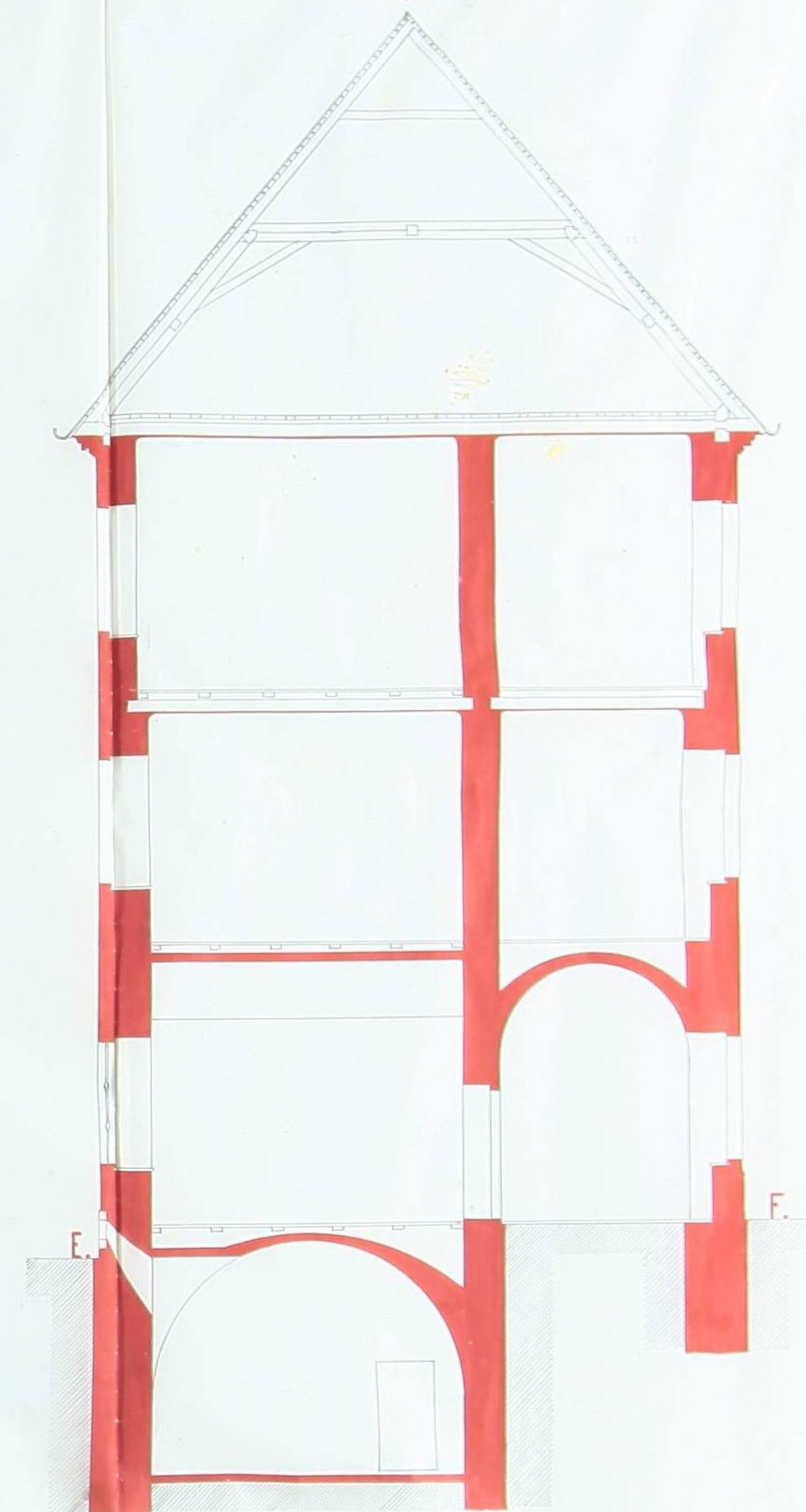
Profil E.F.
