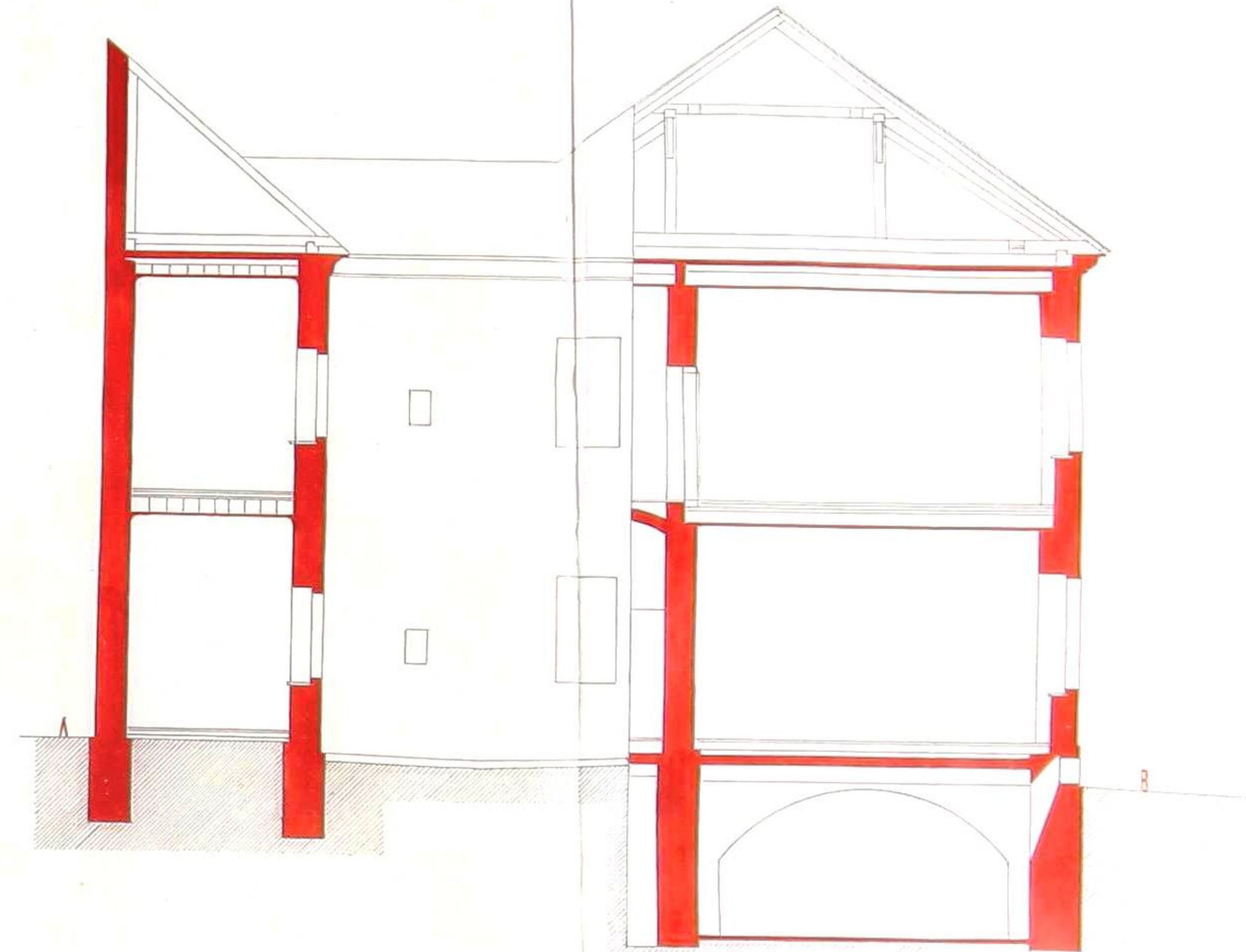
Profil AB.
