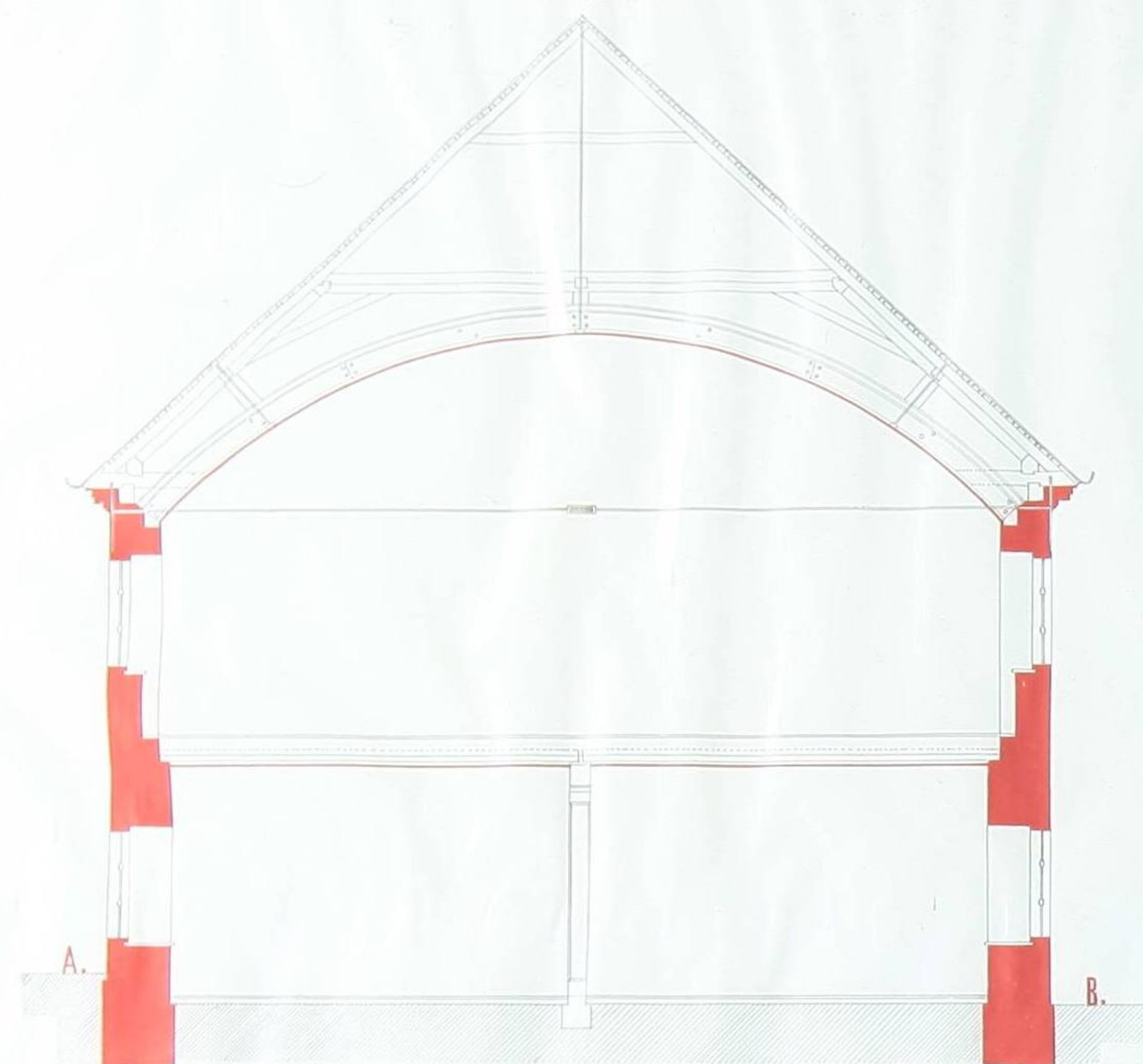
Profil A.B.
