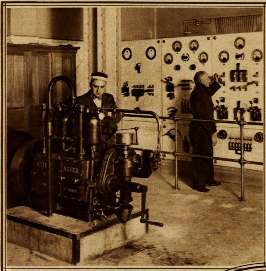
Grupo electrógeno y cuadro de carga.
