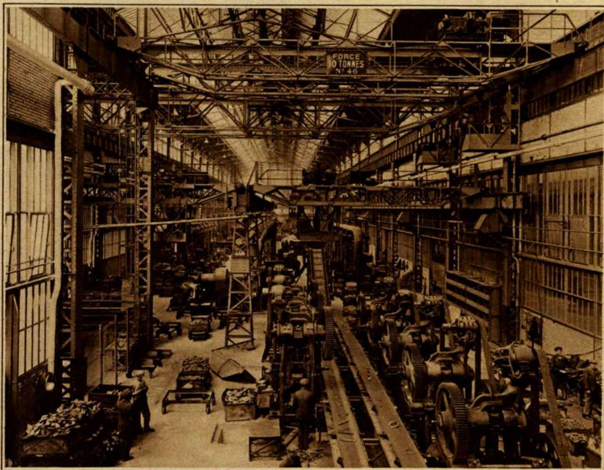
Las máquinas, perfectísimas, van fabricando automáticamente las diferentes piezas que un transportador mecánico remite a los talleres de montaje.
