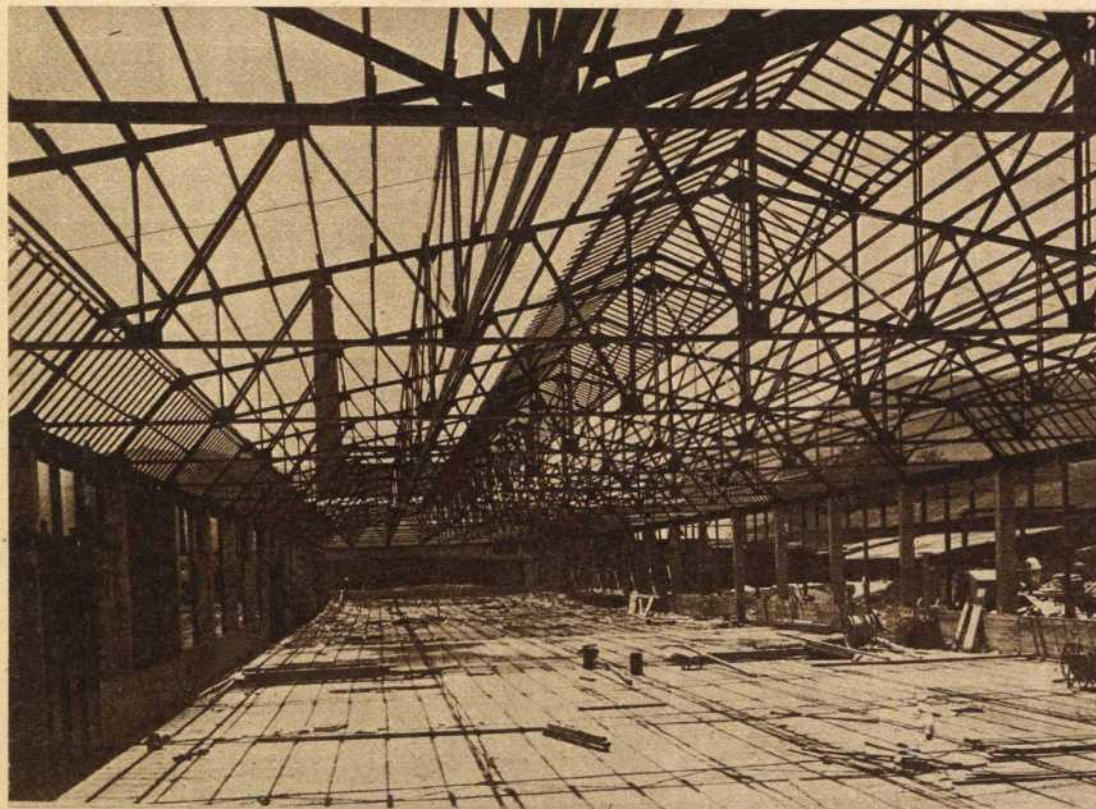
La nueva fábrica de automóviles que se está construyendo en Zorroza (Bilbao) por la S. E. I. D. A., Sociedad Anónima
