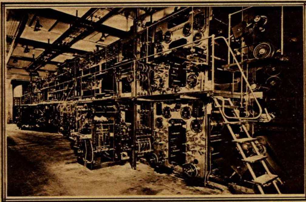
La máquina Winkler que acaba de ser montada para las ediciones de «El Día Gráfico» , «La Noche» y «La Gaceta Deportiva» .
