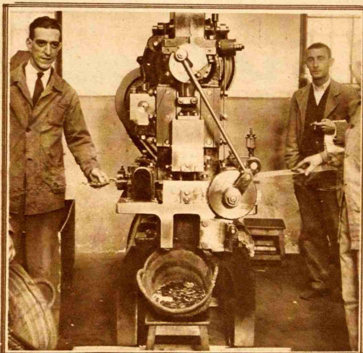
De la plancha se van cortando los discos destinados a convertirse en moneda.
