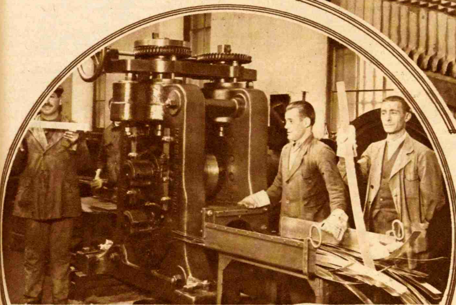
El lingote que sale del molde de fundición se convierte en la plancha de la que se corta la moneda.
